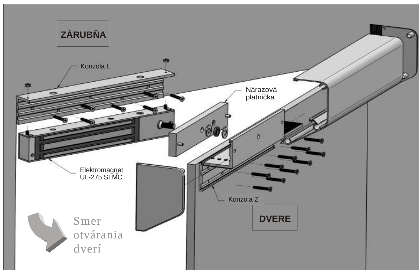
Obrázok 1. Schématický Pohľad
