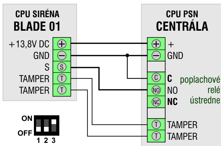
AKTIVÁCIA PRIPOJENÍM ⊖ PÓLU
