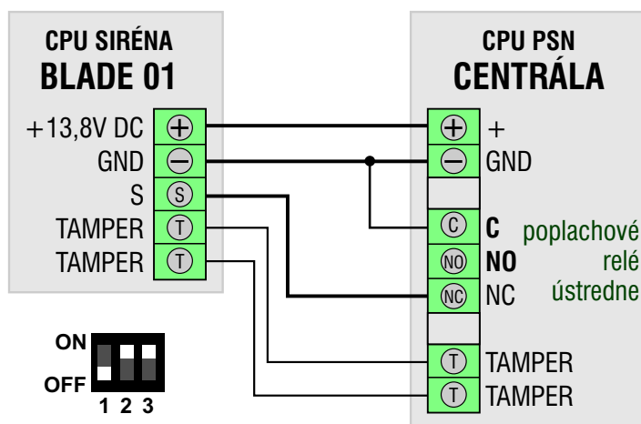
AKTIVÁCIA ODPOJENÍM ⊖ PÓLU
