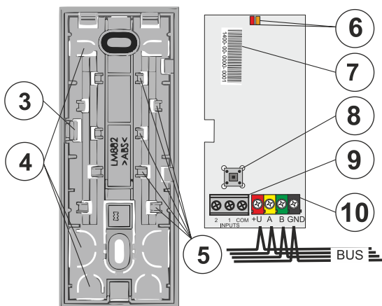
Obr. 2: 3 – západka elektroniky; 4 – vylamovacie prechody; 5 – fixačné príchytky pre káble prichádzajúce z horných prechodov; 6 – červená a žltá kontrolka; 7 – sériové číslo; 8 – sabotážny kontakt; 9 – svorky na pripojenie magnetických detektorov; 10 – svorky zbernice;
