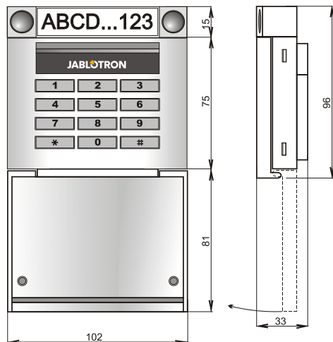
Obr. 5: Rozmery modulu
