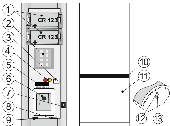
Obr. 1: 1 – držiak batérií, 2 – MW senzor, 3 – konektor pre pripojenie sabotážneho kontaktu klbového držiaka JA-191PL, 4 – LED kontrolky na indikáciu stavu detektora, 5 – sériové číslo, 6 – PIR senzor, 7 – sabotážny kontakt, 8 – anténa, 9 – západka elektroniky, 10 – svetlovod, 11 – šošovka PIR senzora, 12 – otvor pre aretačnú skrutku, 13 – západka krytu
